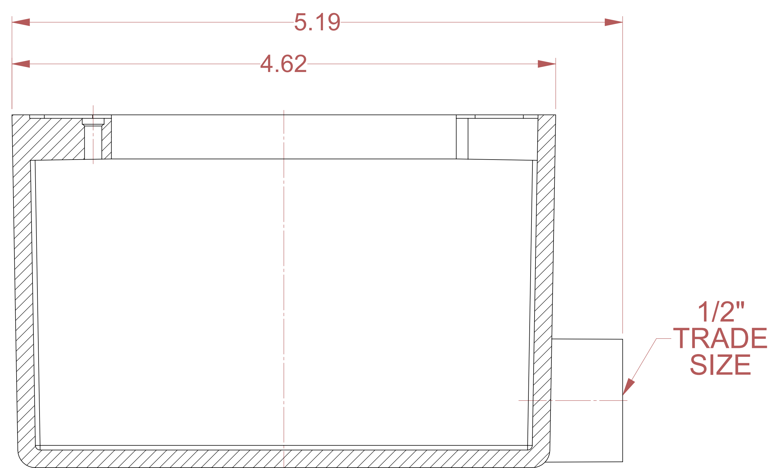
SECTION A-A
