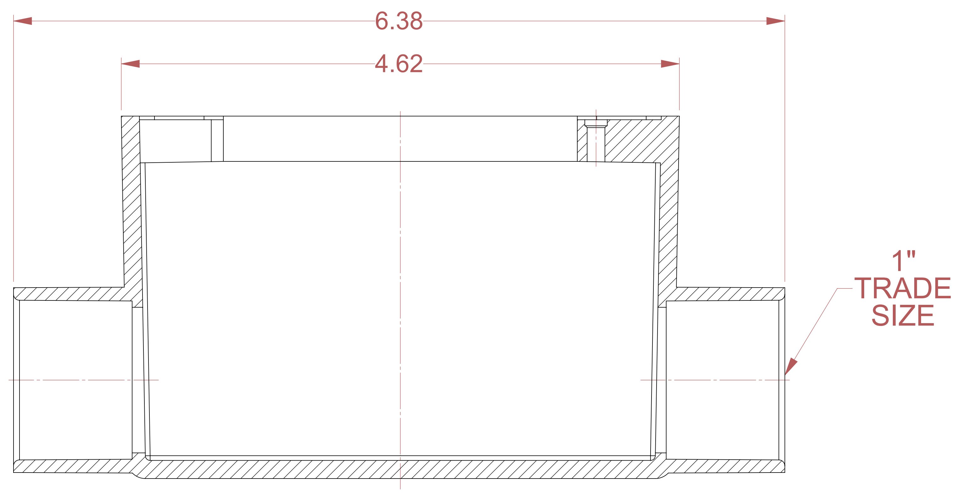
SECTION A-A
