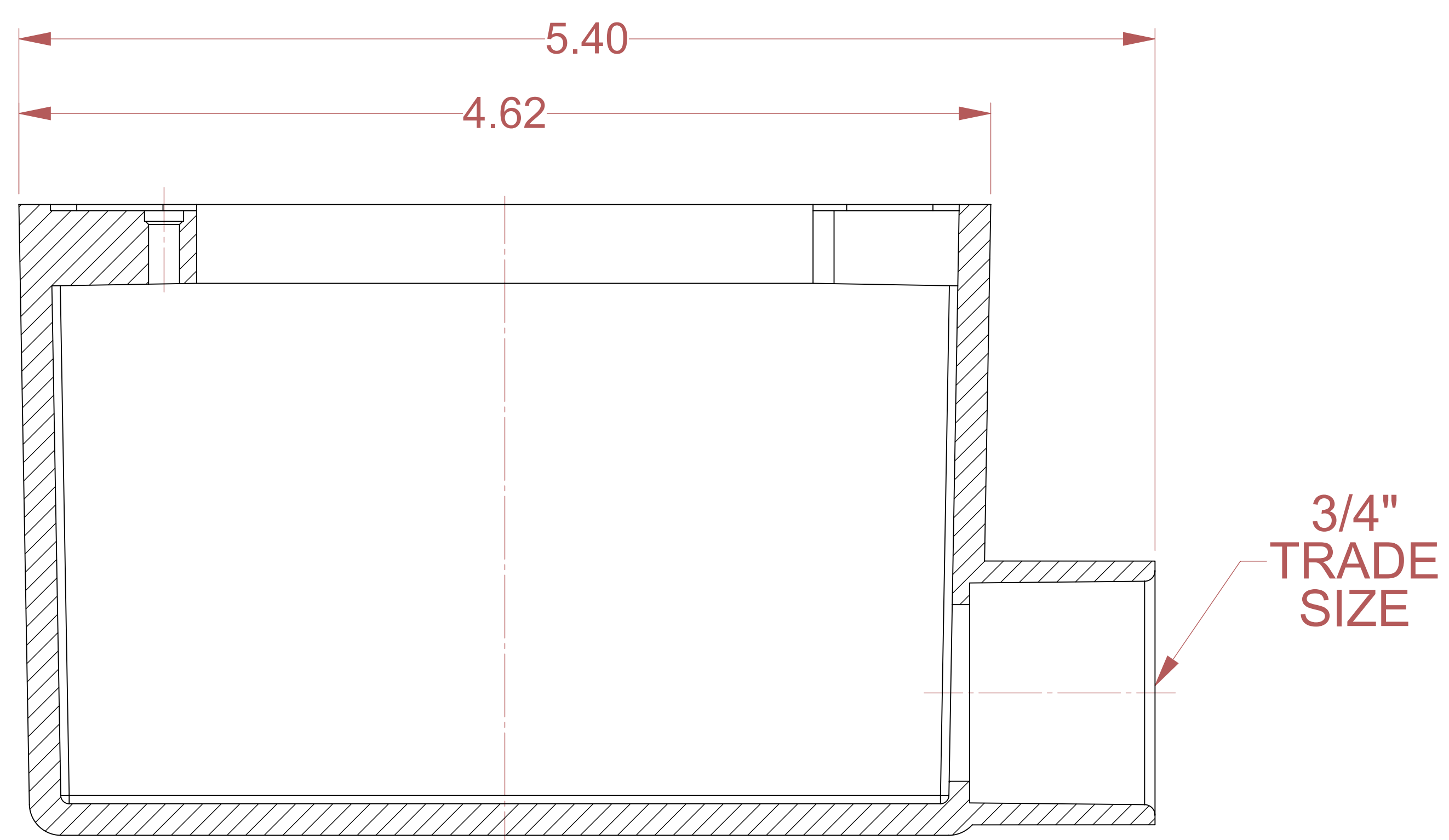
SECTION A-A
