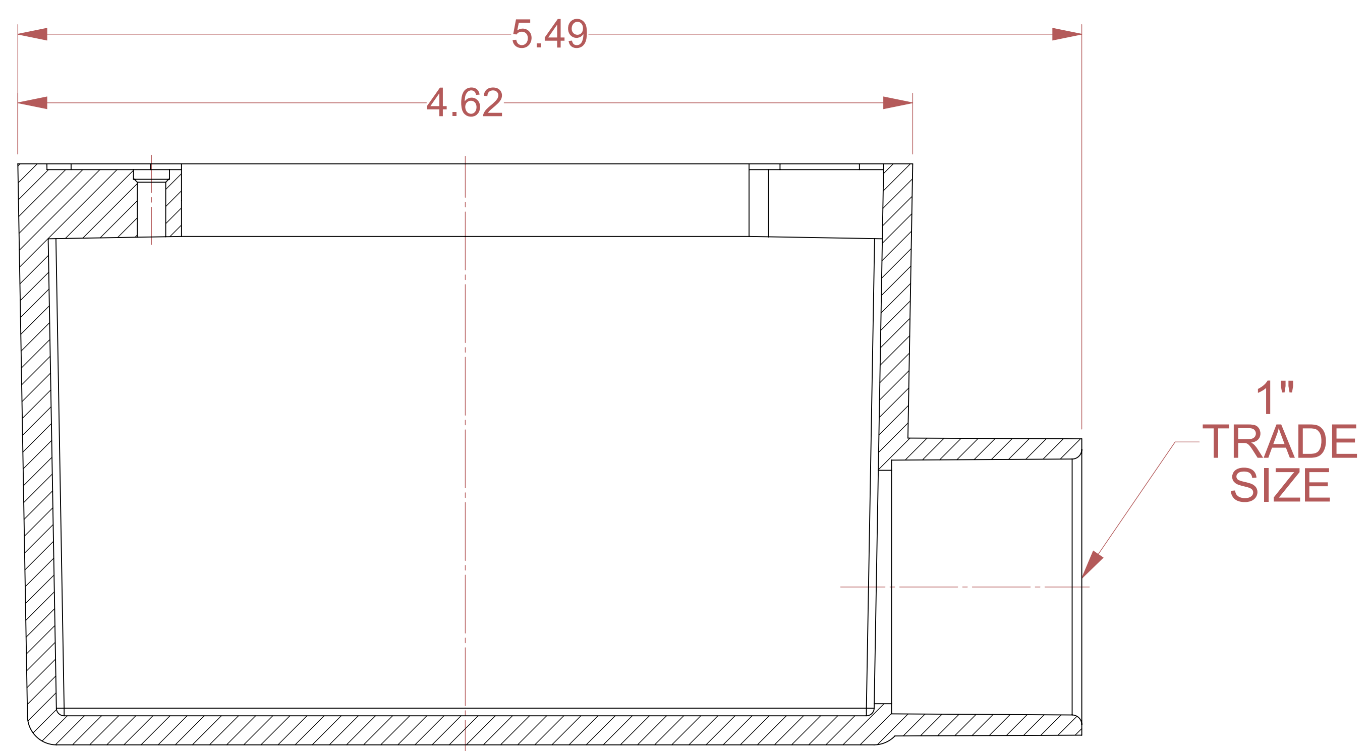
SECTION A-A
