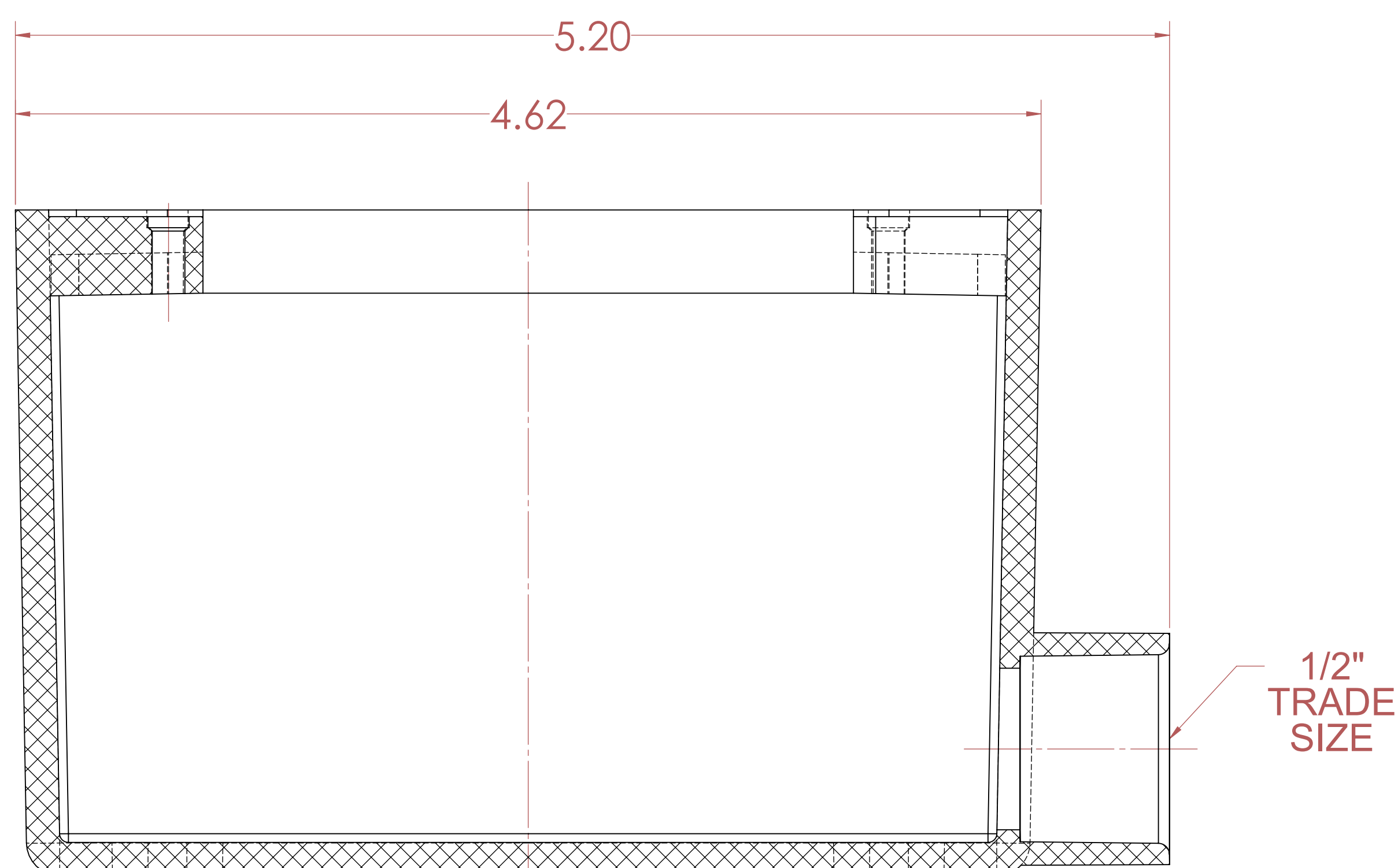
SECTION A-A SCALE 2 : 1
