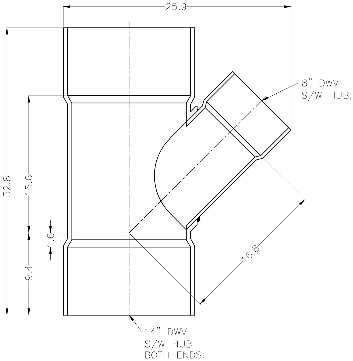
DWV 45 WYE 14X14X8
